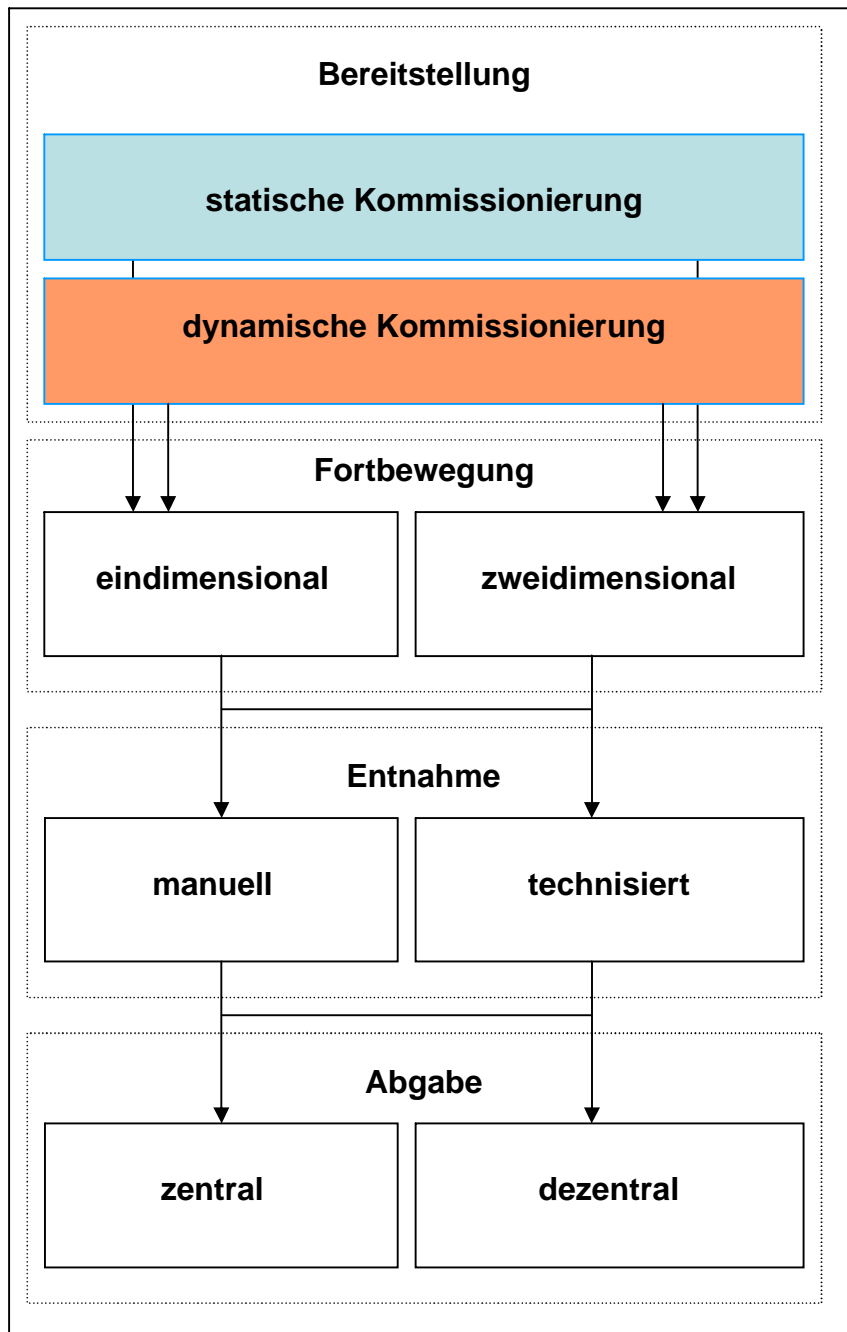
Bild 11.20: Klassifizierung von Kommissioniersystemen aus technischer Sicht
